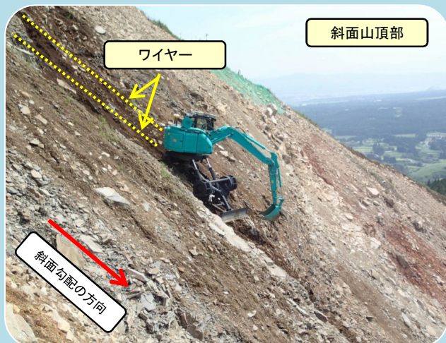
斜面中腹崩壊土除去工状況写真①
